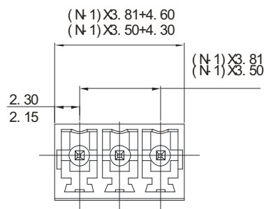
15EDGVC-3.5 15EDGVC-3.81
